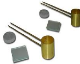
Le Chatelier Mould
